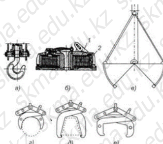
1-электромагнит; 2 — каркас; а-крюк; б-электромагнитная шайба; в-грейфер; г, д, е — зажимные зажимы для валов, отливок и обмоток Рисунок 12.1-грузозахватные устройства
