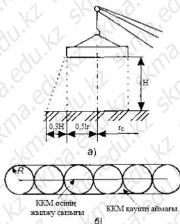
Рисунок 12.1-схема определения опасной зоны в грузоподъемном механизме
